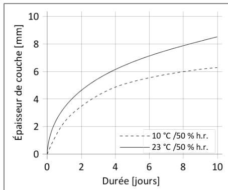
Diagramme 1: Vitesse de durcissement de Sikaflex®-552 AT
