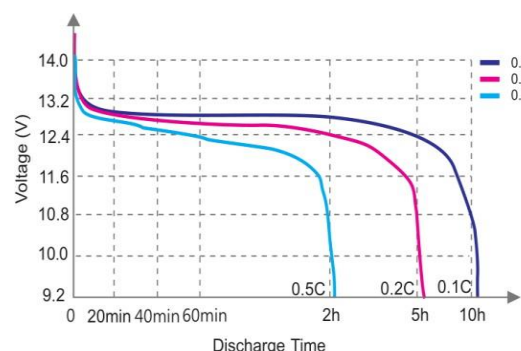
Courbes de décharge de différents courants
