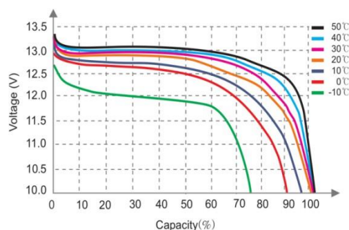
Courbes de décharge à différentes températures
