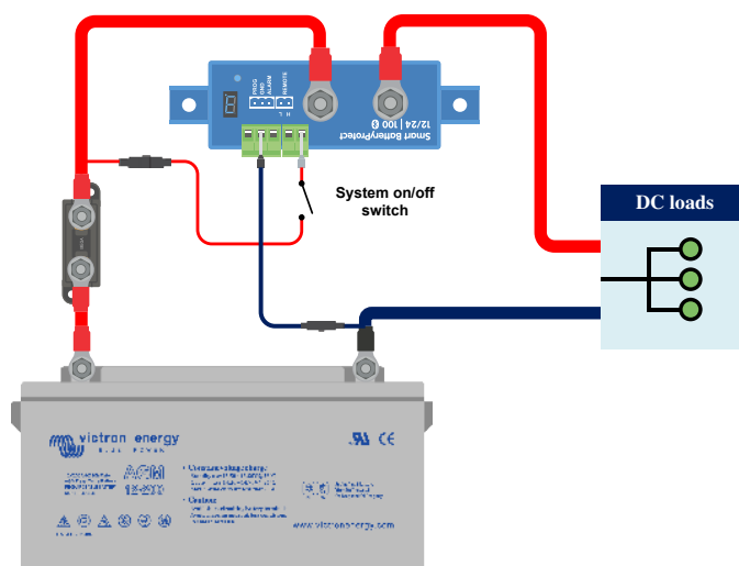
Interrupteur câblé entre le positif de la batterie et l'entrée H de la borne à distance
